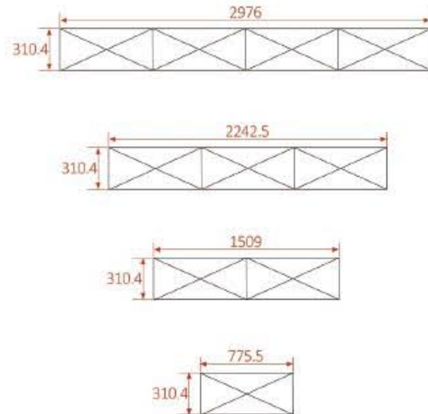
LT-09L2-A Square Tube Frame
